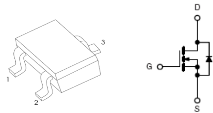
SOT - 523
