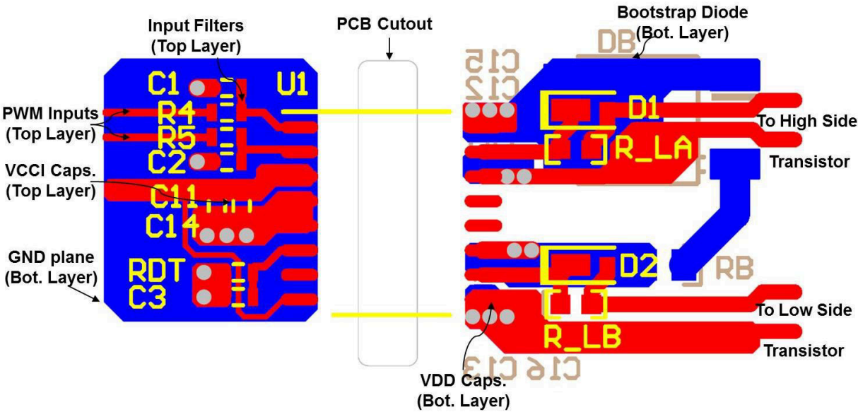
图 11-1. 布局示例
