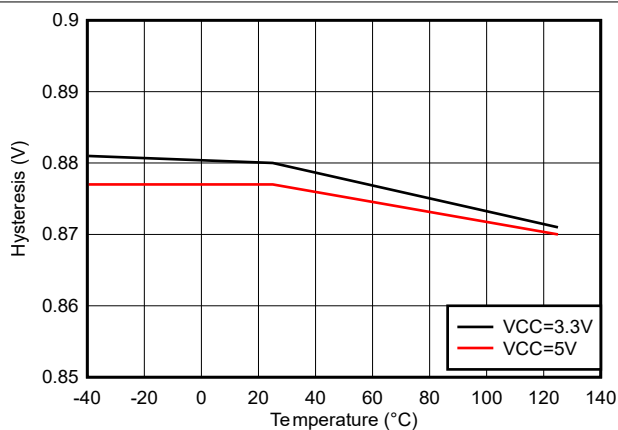
图 5-21. IN/DIS 迟滞与温度之间的关系
