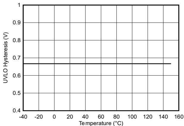
图 5-19. VDD 8V UVLO 迟滞与温度之间的关系
