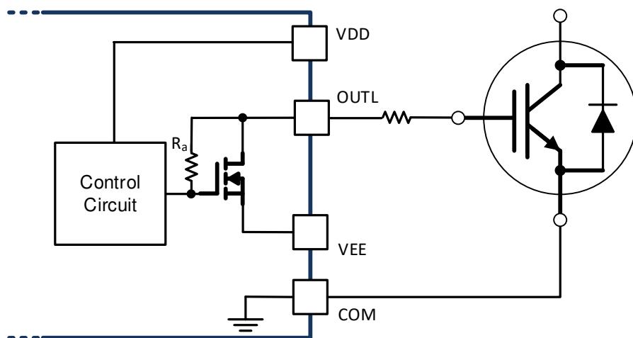
图 8-2. Active Pulldown
