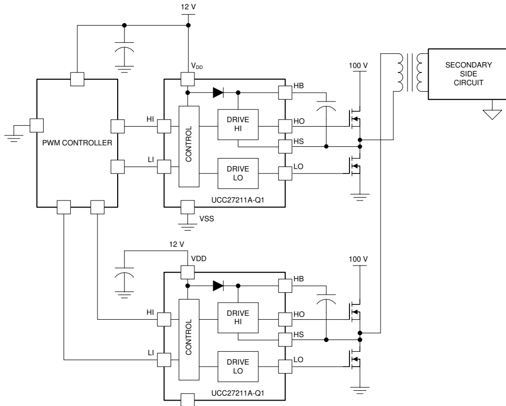
图 7-2. UCC27211A-Q1 典型应用图 2
