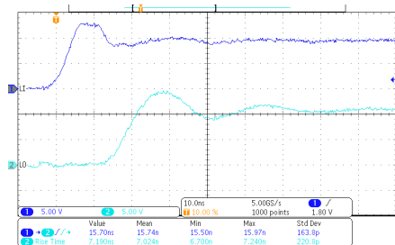
图 7-3. LO 上升时间和 LI 至 LO 导通传播延迟
