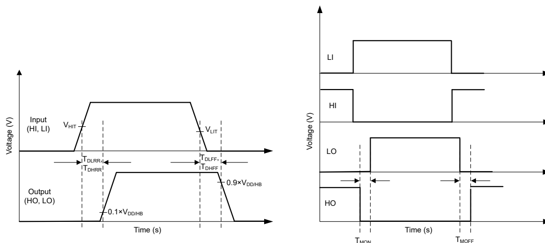
图 5-1. 时序图
