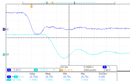
图 7-4. LO 下降时间和 LI 至 LO 关断传播延迟
