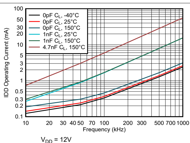
图 5-3. I_{DD} 工作电流与频率间的关系
