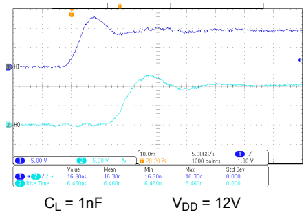
图 7-5. HO 上升时间和 HI 至 HO 导通传播延迟
