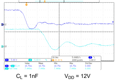
图 7-4. LO 下降时间和 LI 至 LO 关断传播延迟
