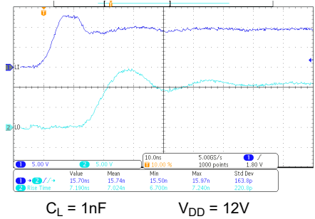
图 7-3. LO 上升时间和 LI 至 LO 导通传播延迟
