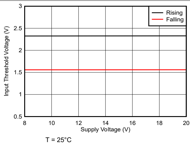
图 5-5. 输入阈值与电源电压间的关系
