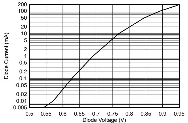
图 5-15. 二极管电流与二极管电压间的关系
