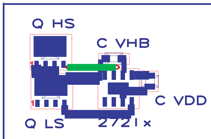
图 7-7. UCC27211 元件放置
