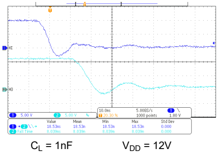
图 7-6. HO 下降时间和 HI 至 HO 关断传播延迟
