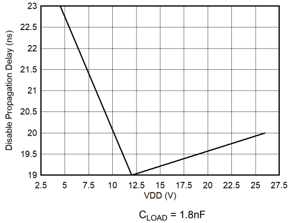
图 6-21. 使能到输出下降传播延迟
